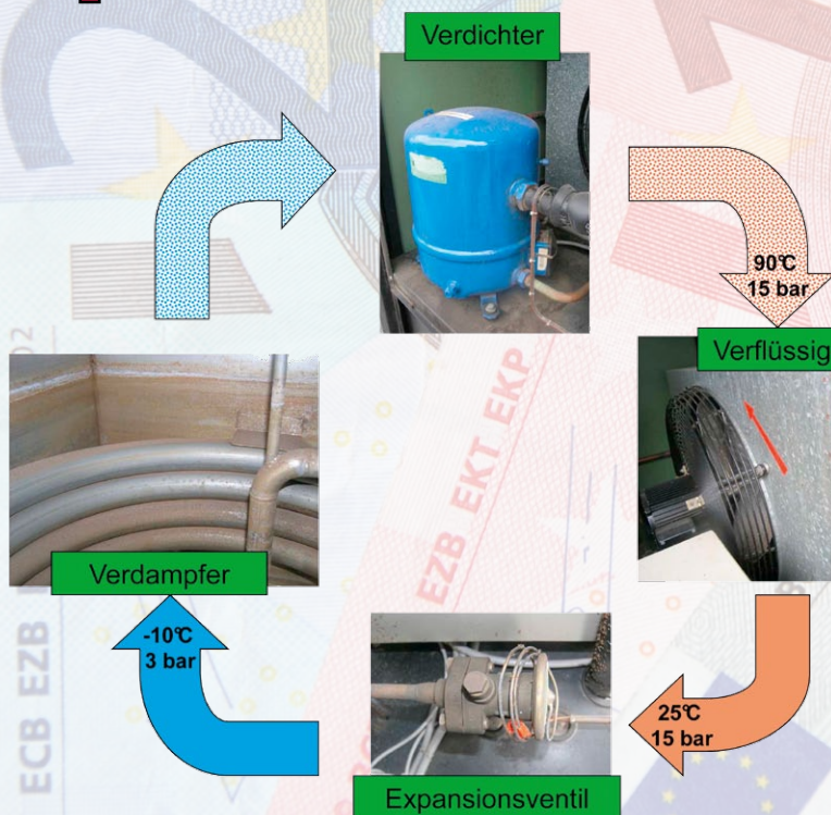
Abb. 1: Aufbau einer Kältemaschine am winzerüblichen Beispiel eines Kühlwasserrückkühlgerätes
